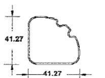
PERFIL TRIANGULAR CURVO RANURADO (PATA)
