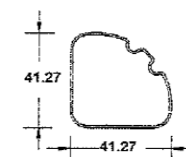
PERFIL TRIANGULAR CURVO RANURADO (PATA)
