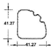
PERFIL TRIANGULAR CURVO RANURADO (PATA)
