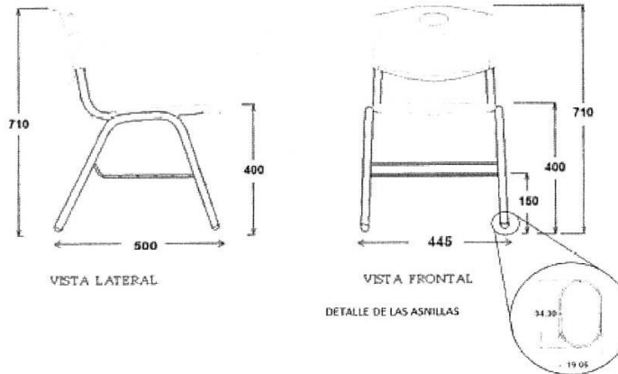
SILLA PARA MESA BINARIA DE 4° A 6°
