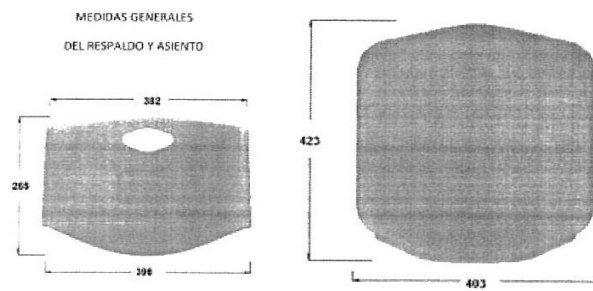
SILLA PARA MESA BINARIA DE 4° A 6°
