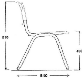
SILLA PARA MAESTRO
