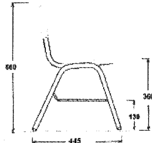
VISTA LATERAL
