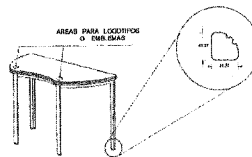
MESA PARA SILLA BINARIA DE 4" A 6"
