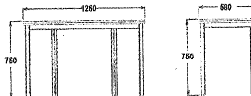
MESA PARA SILLA BINARIA DE 4" A 6"
