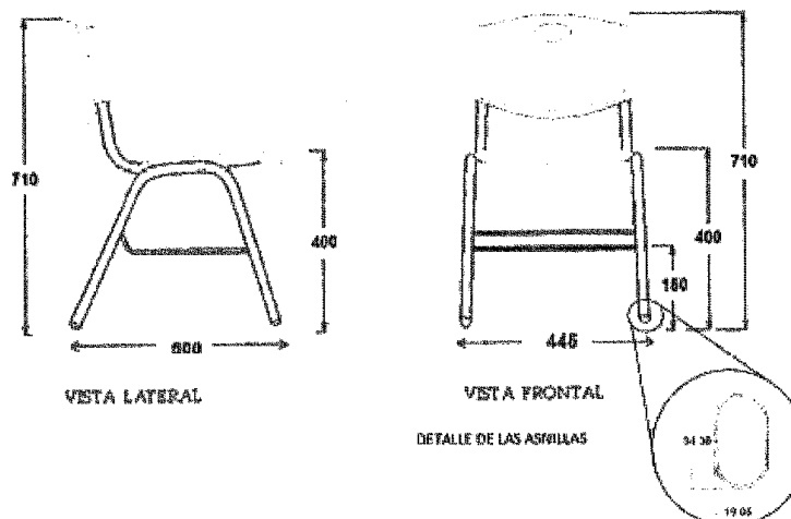
SILLA PARA MESA BINARIA DE 4° A 6°
